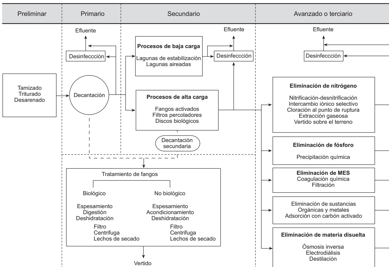
Figura 42.1. Diagrama del flujo general del proceso de tratamiento del agua residual.
