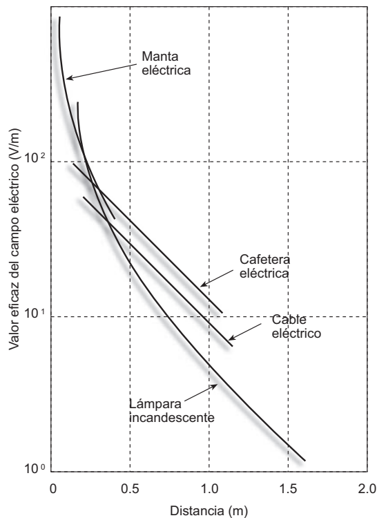
Figura 40.5. Campos eléctricos producidos por aparatos comunes en las casas en función de la distancia.
