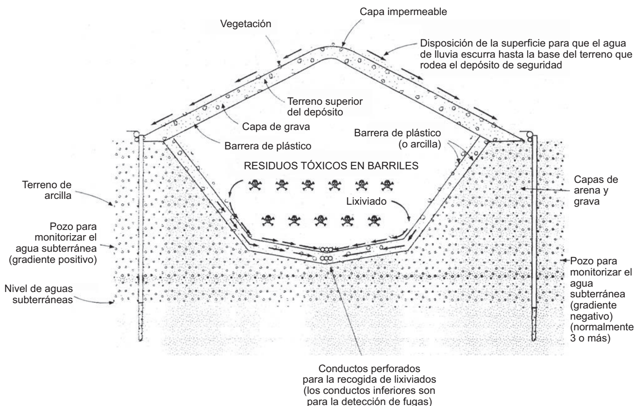
Figura 43.10. Depósito de seguridad de los RP.
