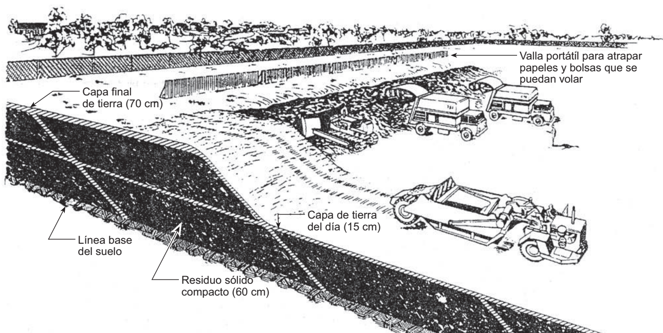
Figura 43.4. Vertedero controlado. El camión deposita una carga de residuos sólidos. El tractor oruga los nivela y los compacta. Finalmente, la excavadora de arrastre (en primer plano), transporta el material de cobertura al final de las operaciones cotidianas. Puede observarse la existencia de una rejilla portátil para atrapar los plásticos y papeles, y otras partículas volantes. Estas rejillas deben emplearse siempre que resulten necesarias.
