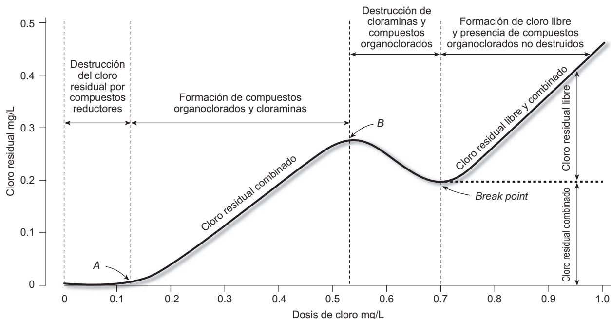
Figura 41.5. Cloración al punto de ruptura.
