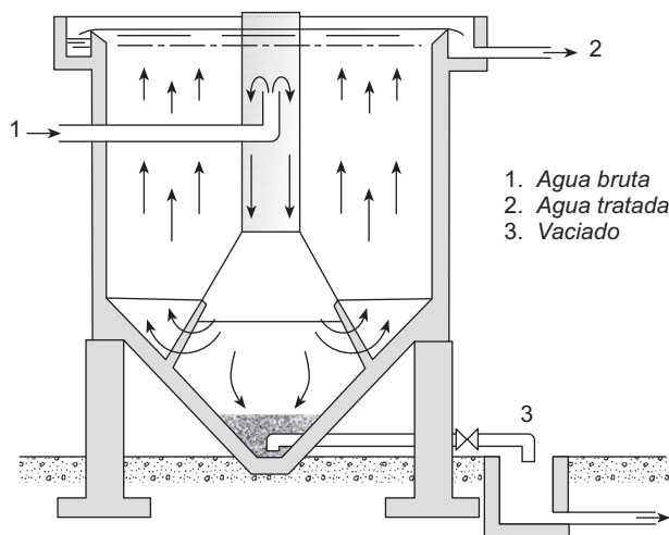
Figura 41.2. Decantador cilindro-cónico.
