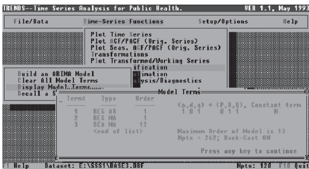
Figura 36.27. Parámetros del ajuste del modelo ARIMA para una serie temporal.
