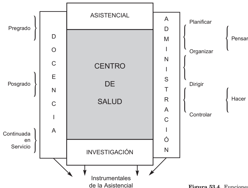
Figura 53.4. Funciones del Personal Sanitario.
