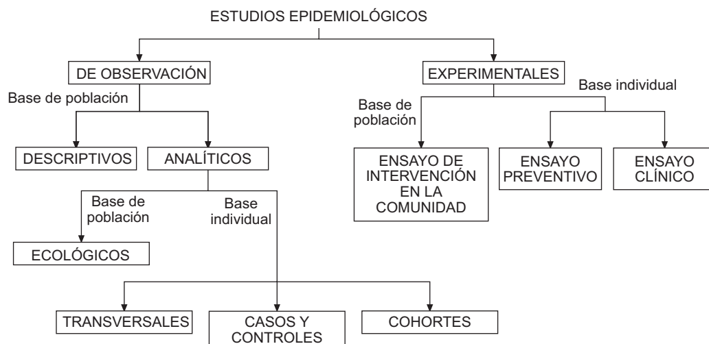
Figura 29.1. Tipos de estudios epidemiológicos.
