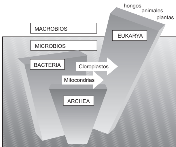
Figura 39.1. Clasificación de los seres vivos: los 3 dominios.
