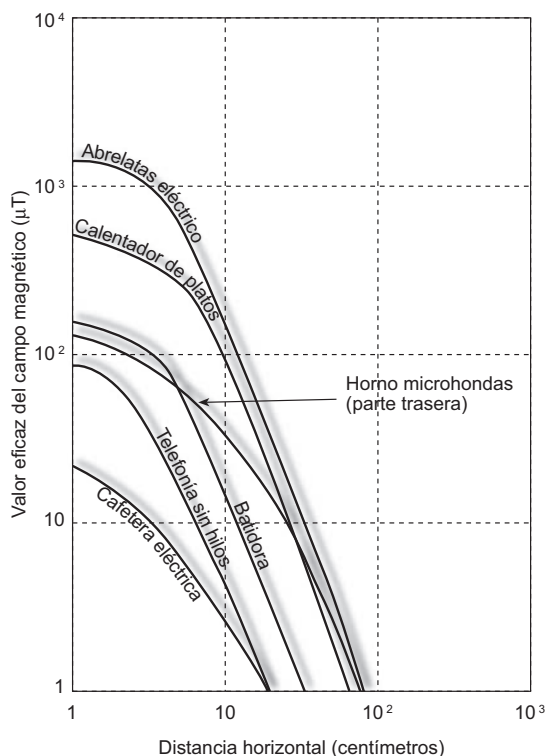
Figura 40.6. Valores de campos magnéticos generados por distintos aparatos electrodomésticos en función de la distancia.
