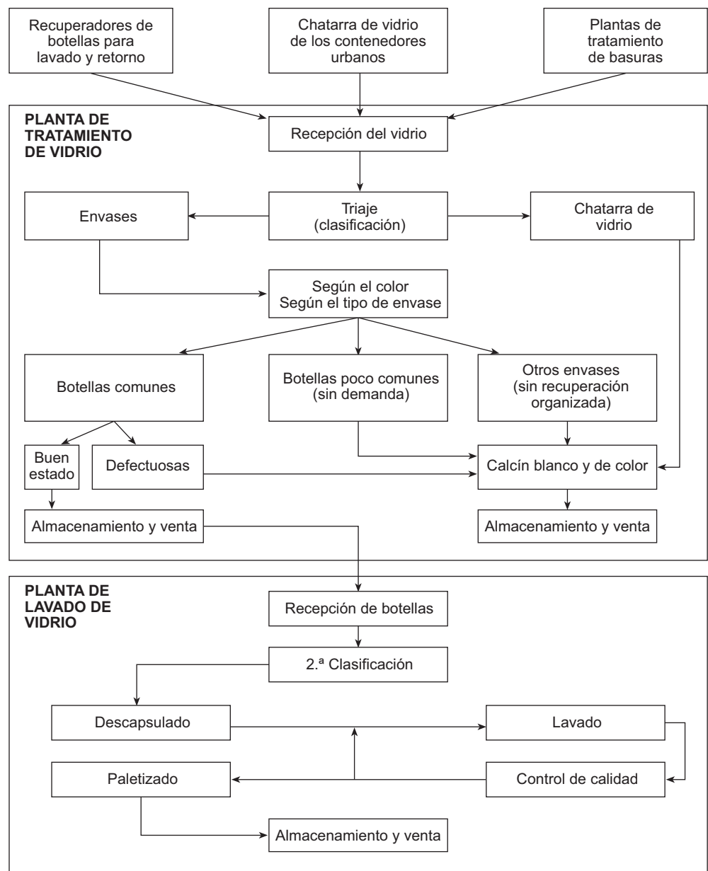
Figura 43.6. Esquema del proceso de recogida del vidrio.
