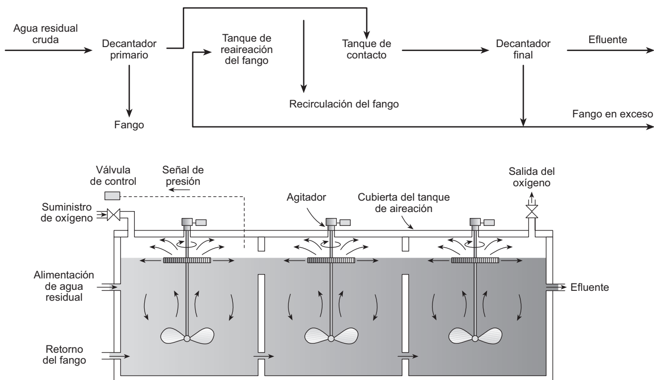
Figura 42.3. Diagrama de flujo para el proceso de fangos activados de contacto y estabilización, y detalle del tanque de contacto.
