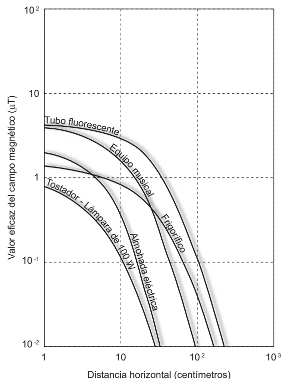
Figura 40.6. Valores de campos magnéticos generados por distintos aparatos electrodomésticos en función de la distancia.
