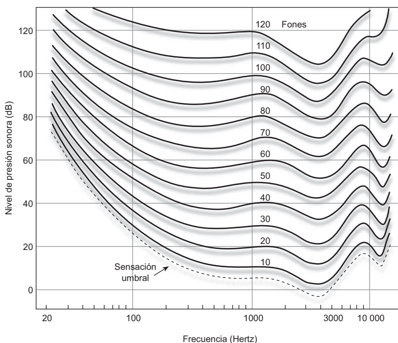
Figura 40.1. Curvas de sensación del sonido.
