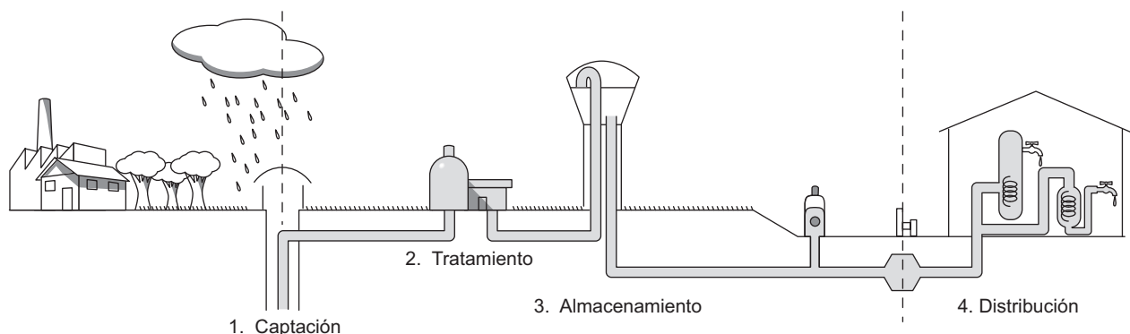
Figura 41.1. Esquema de un sistema de abastecimiento.
