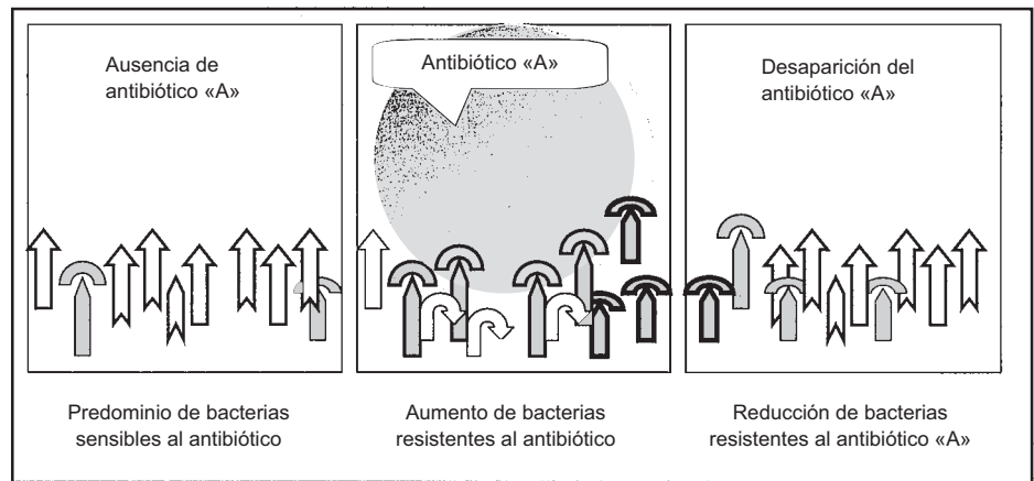
Figura 39.7. Ciclo temporal de la resistencia bacteriana a los antibióticos.
