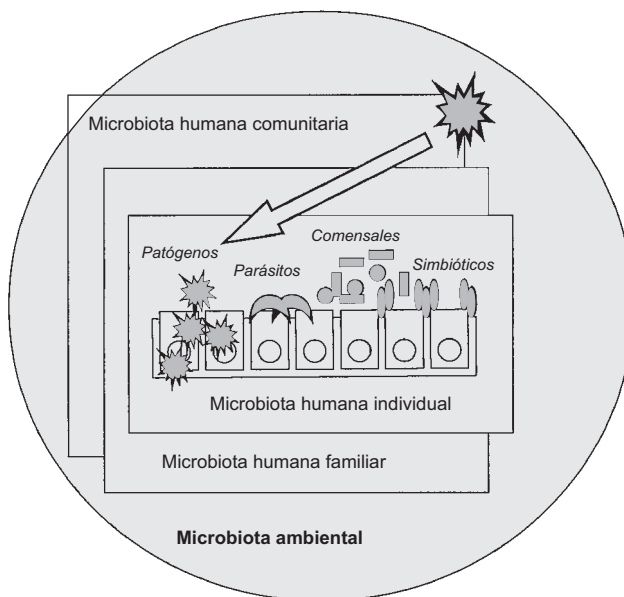
Figura 39.6. Microbiota humana y ambiental.
