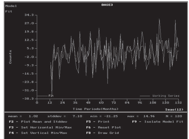
Figura 36.28. Serie temporal y de ajuste del modelo ARIMA.
