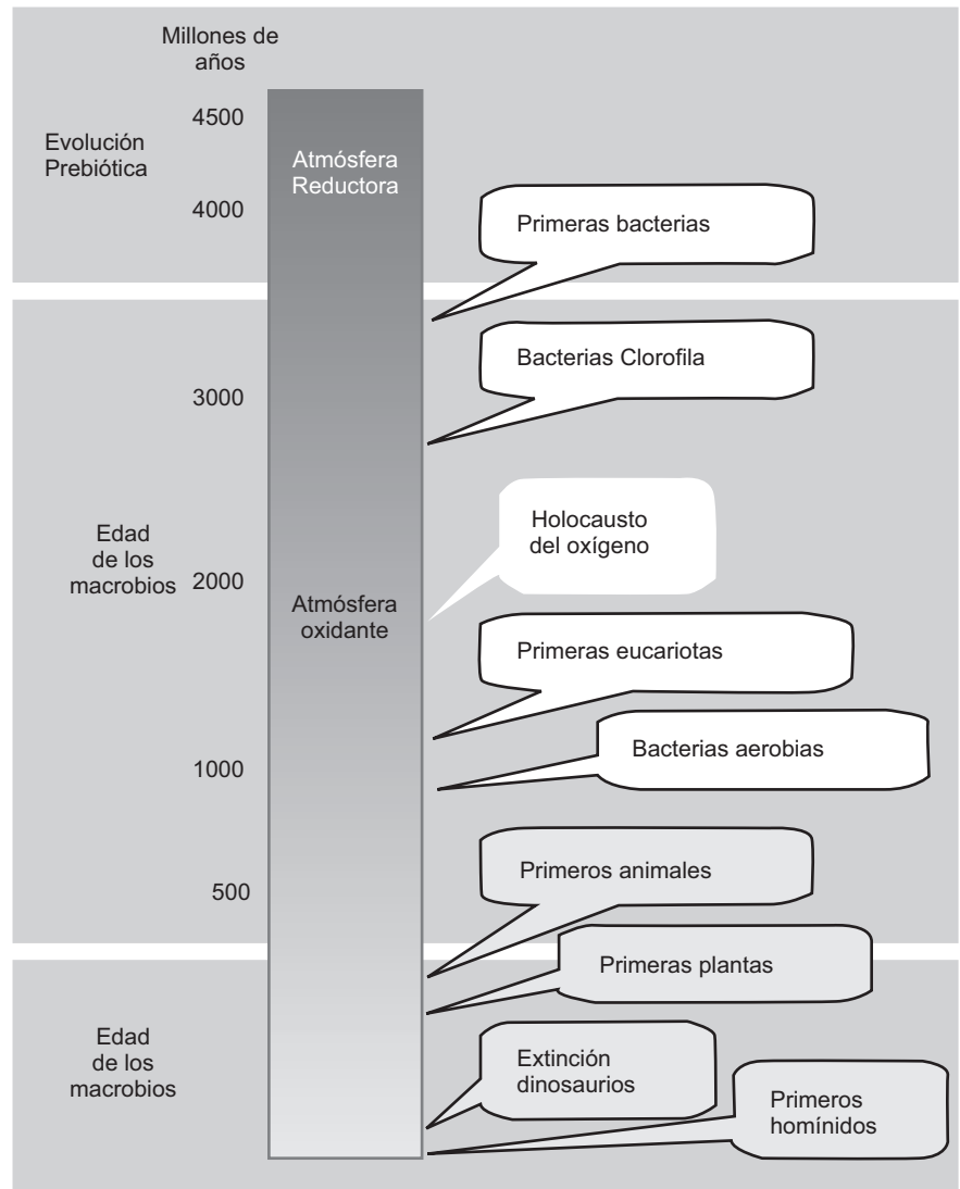
Figura 39.2. Evolución de la vida en el planeta.
