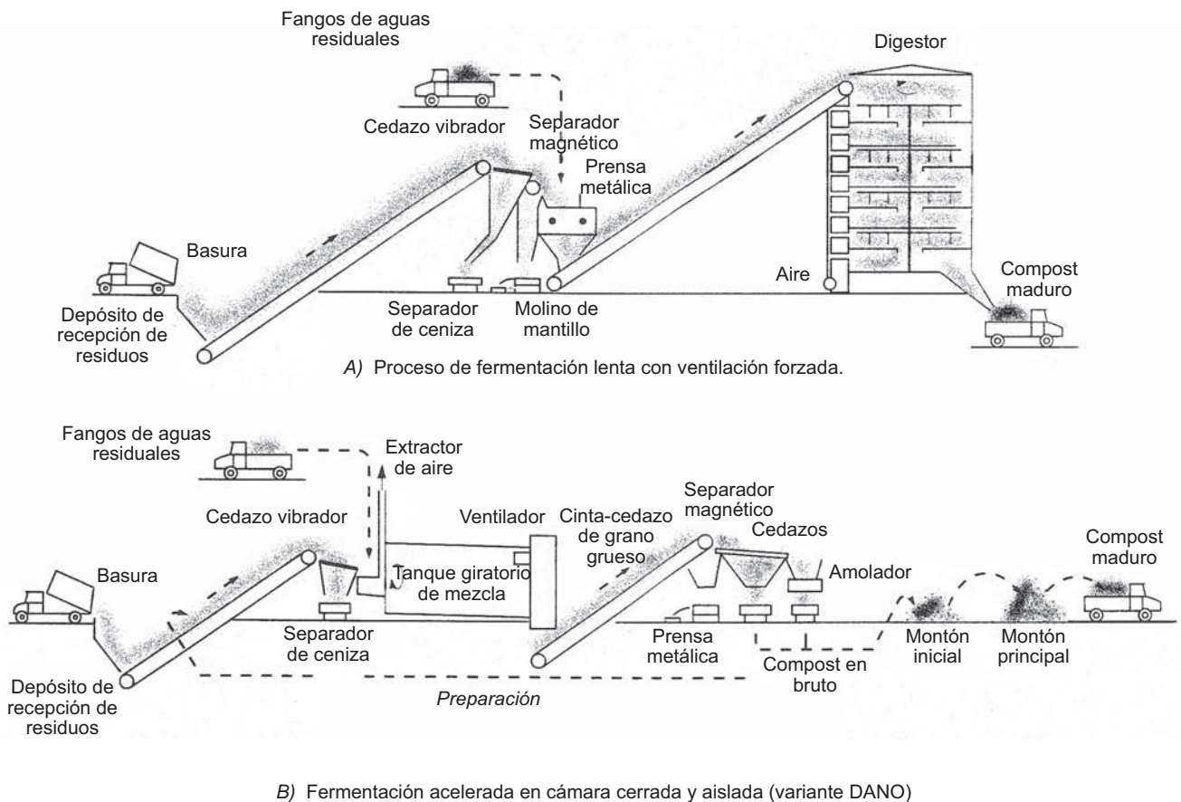
Figura 43.8. Operaciones mecanizadas para obtener compost.
