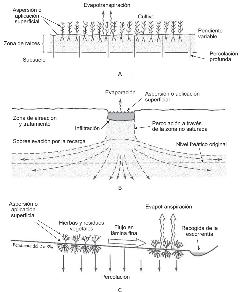
Figura 42.4. Los tres procesos principales de aplicación al terreno: A) regadío. B) infiltración rápida. C) circulación superficial en lámina (escorrentía superficial).
