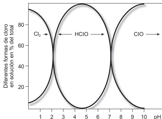
Figura 41.4. Reacciones del cloro con el agua en función del pH.
