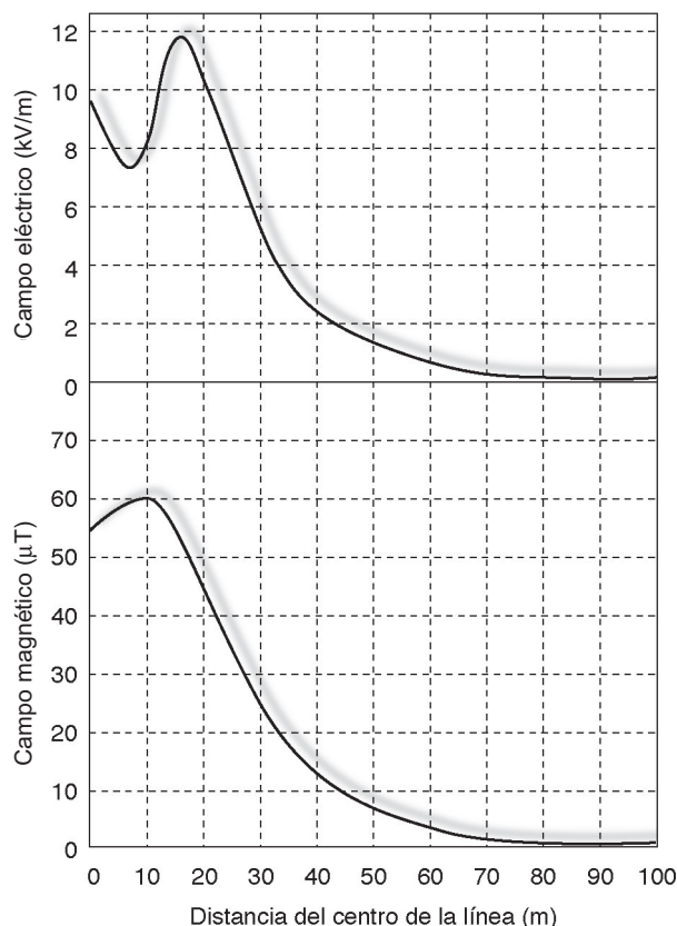
Figura 40.4. Valores típicos de los campos eléctricos (arriba) y magnético (debajo) a nivel de la tierra producidos por una línea de transmisión de 765 kV/m.
